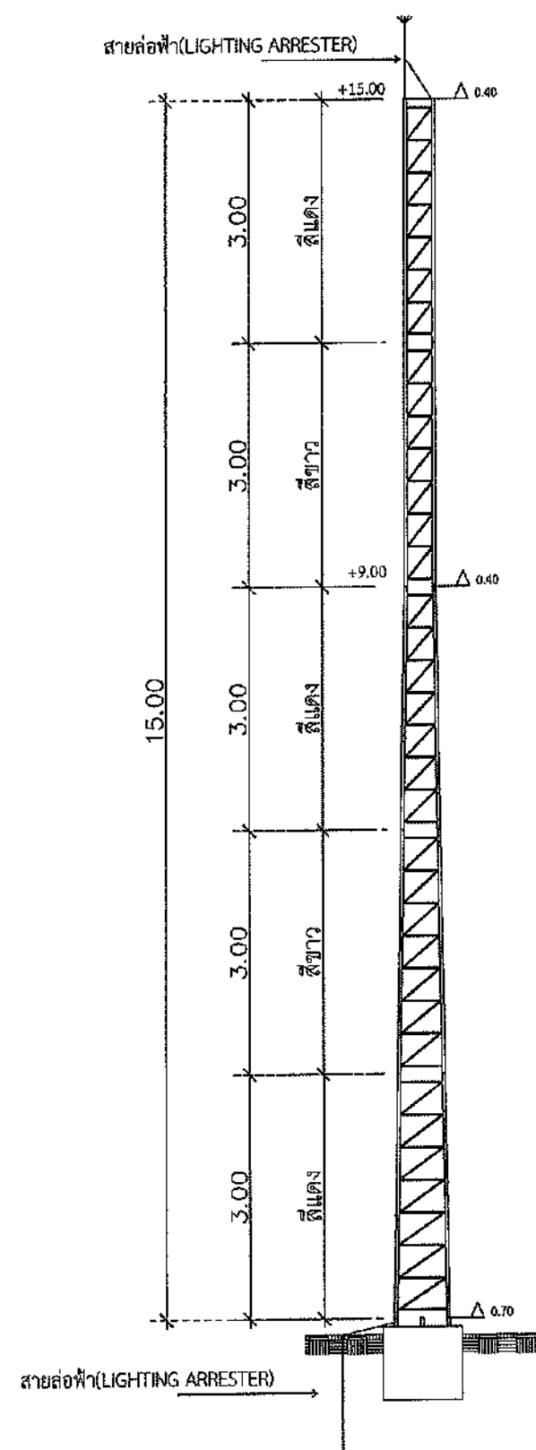
เสาโครงถักลอยตัว SELF - SUPPORT TOWER
