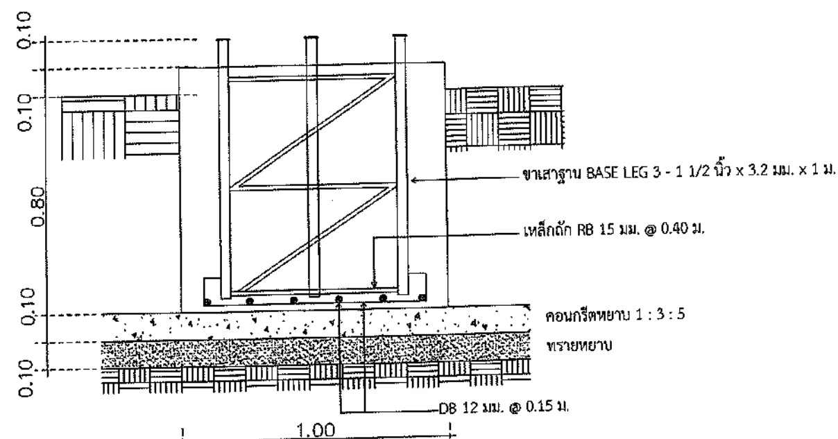
แบบขยายฐานราก FOOTING DETAIL
