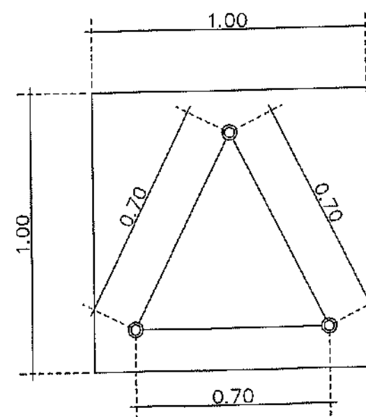
แปลน SELF - SUPPORT TOWER
