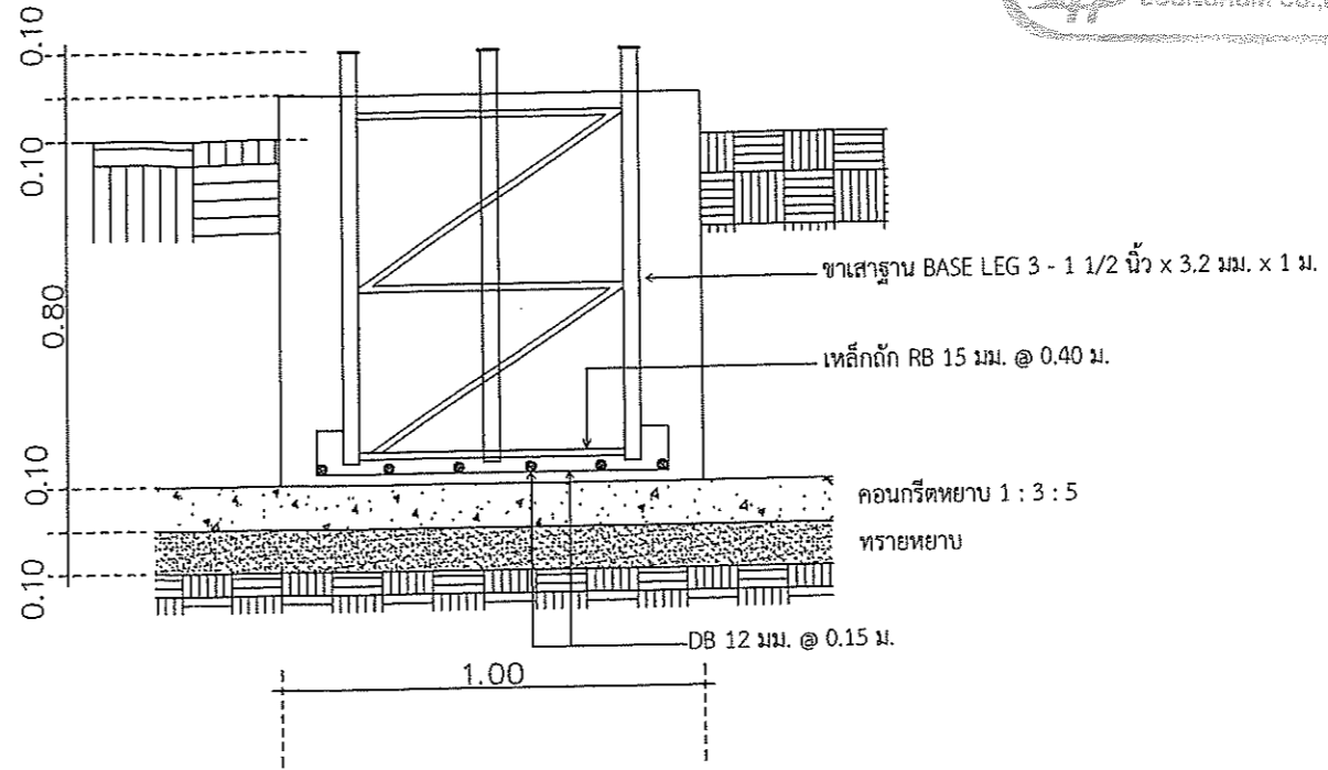
แบบขยายฐานราก FOOTING DETAIL
